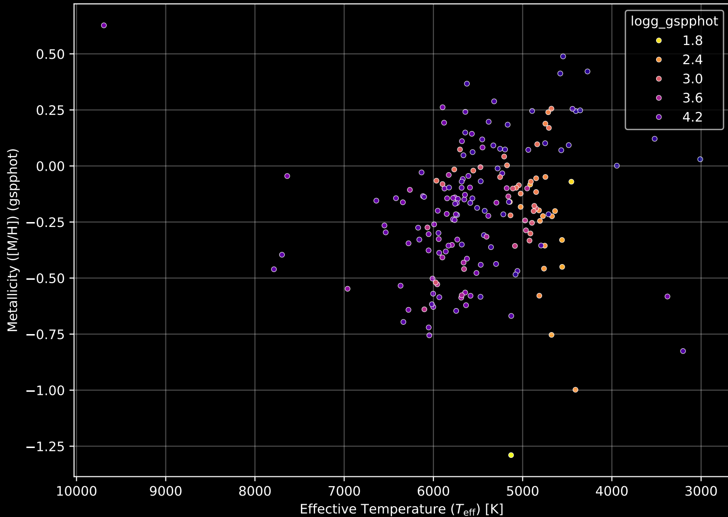
APOGEE DR17 Field: [265-31-O_TESS] Stellar Population Parameters (n= 182)
